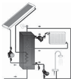
Рис. 10. Система отопления с солнечным коллектором
