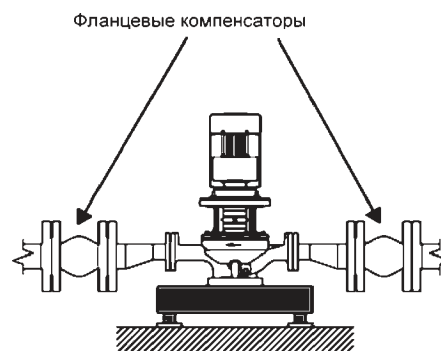
Рис. 30. Насос ТР с фланцевыми компенсаторами увеличенного размера
