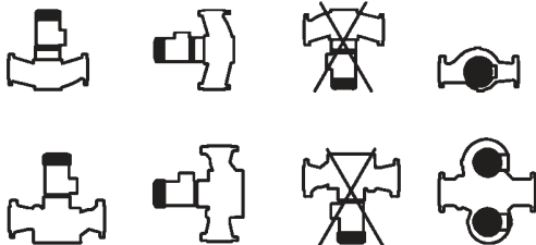
Рис. 23. Монтаж насосов с электродвигателями мощностью менее 11 кВт
