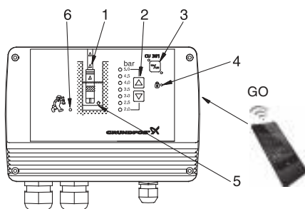
Рис. 22. Блок CU 301 и устройство GO.
