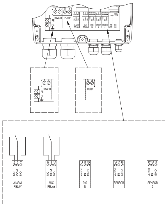
Рис. 32. CU 300 подключение.
