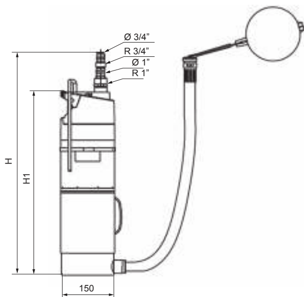
Рис. 45. Модель SBA с поплавковым сетчатым фильтром
