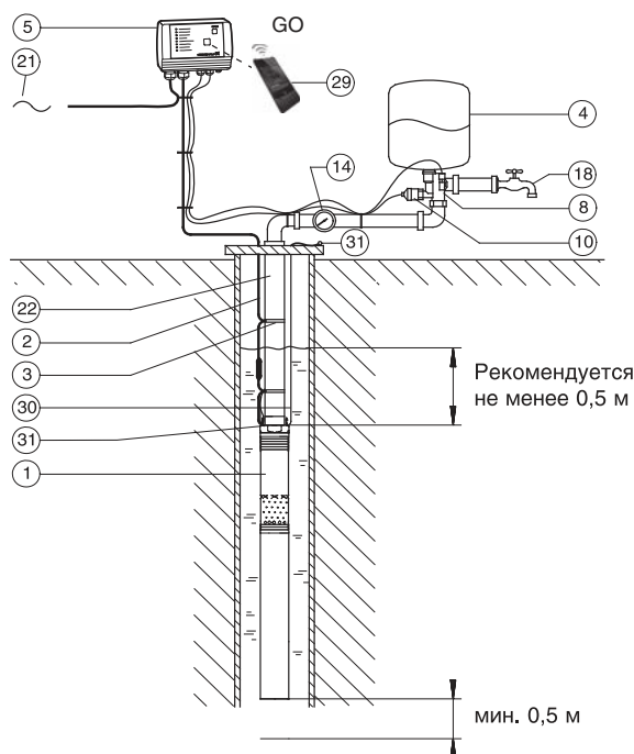
Рис 13. Насос типа SQE и CU 300 в системе водоснабжения (поддержание постоянного давления).
