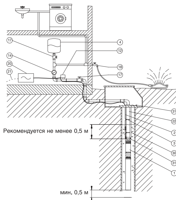
Рис 9. Насос типа SQ в системе водоснабжения частных домов.
