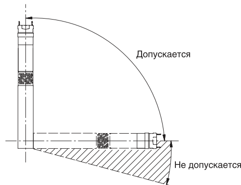
Рис 8. Монтаж насоса SQ/SQE.
