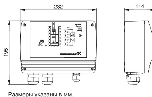
Рис. 24. Блок CU 301 габаритные размеры.
