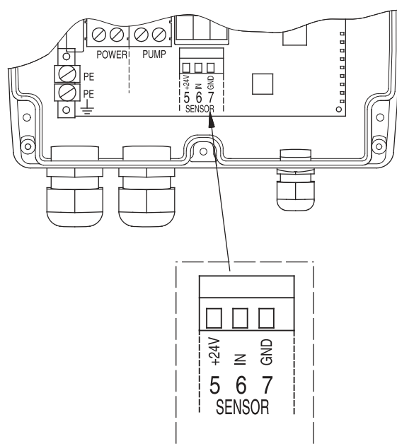
Рис. 33. CU 301 подключение.
