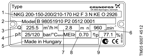
Рис. 5 Пример фирменной таблички
