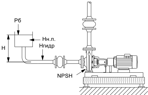
Рис. 41 Высота всасывания воды при отрицательном значении "Н"
