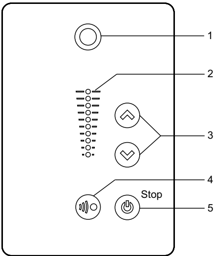
Рис. 58 Панель управления для 2-полюсных электродвигателей 1,1 - 2,2 кВт и 4-полюсных электродвигателей 0,55 - 1,1 кВт
