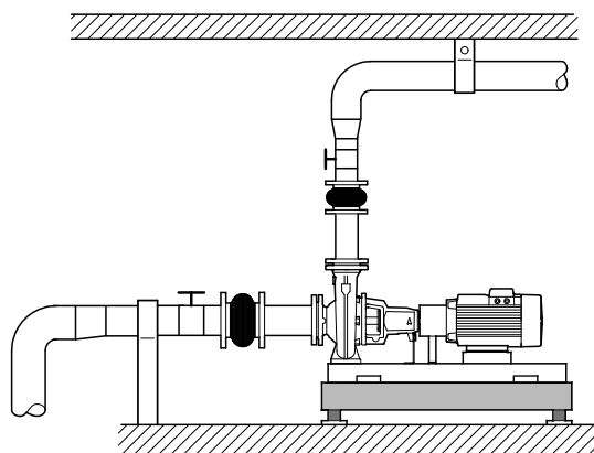
Рис. 49 Монтаж трубопровода
