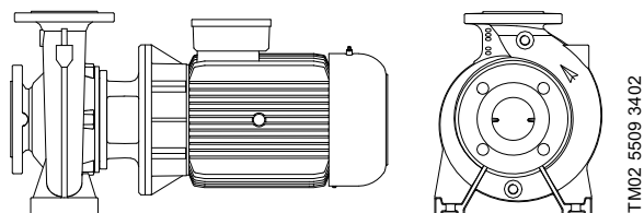
Рис. 16 Исполнение А
