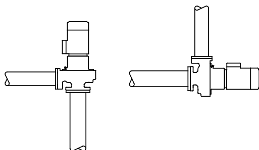
Рис. 50 Прямое соединение насоса с трубопроводом
