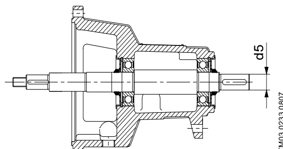
Рис. 21 Фонарь насоса и вал
