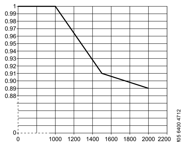
Рис. 36 Максимальная мощность двигателя в зависимости от высоты над уровнем моря
