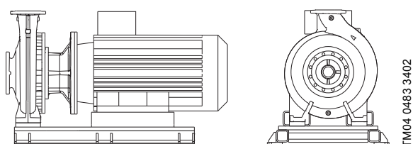
Рис. 19 Исполнение F
