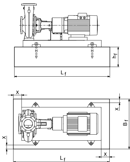
Рис. 42 Фундамент, X \geq \text{мин. } 100 \text{ мм}
