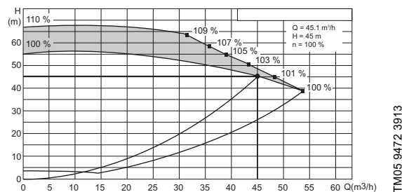
Рис. 54 Расширенный диапазон рабочих характеристик Е-насосов
