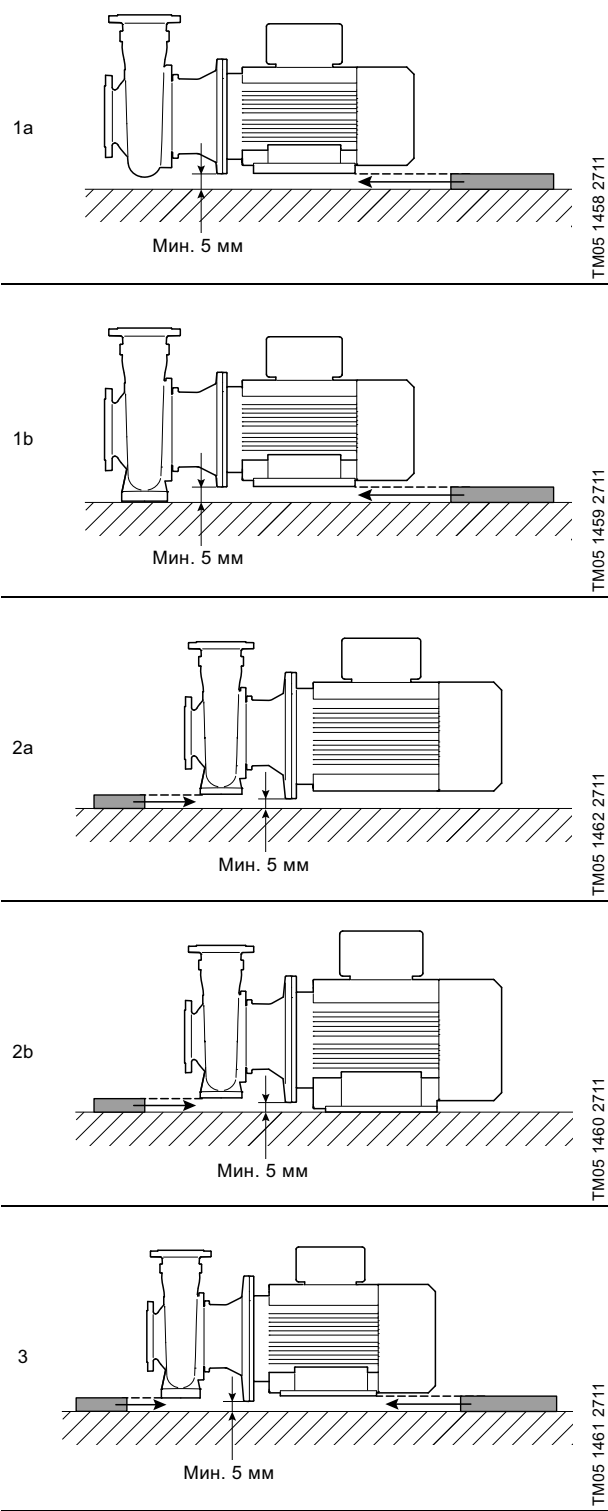
Установочные пластины
