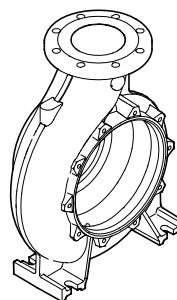
Рис. 20 Корпус насоса NBG и NKG с радиальным отводом
