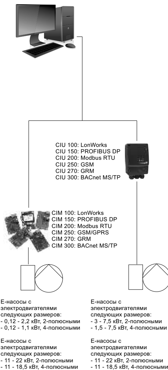
Рис. 61 Схема центральной системы управления зданием
