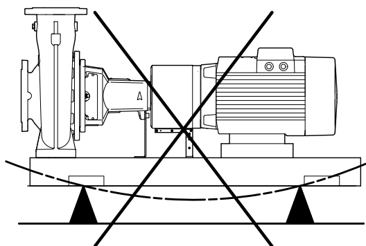
Рис. 44 Неправильный фундамент
