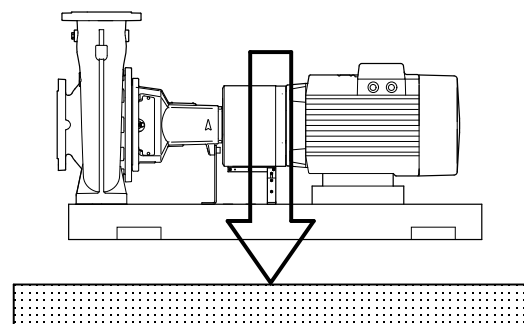
Рис. 43 Правильная установка
