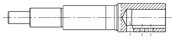
Рис. 25 Вал насоса NBG
