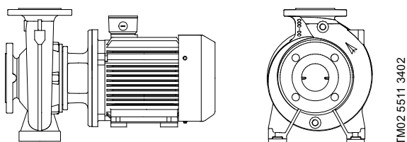
Рис. 18 Исполнение С
