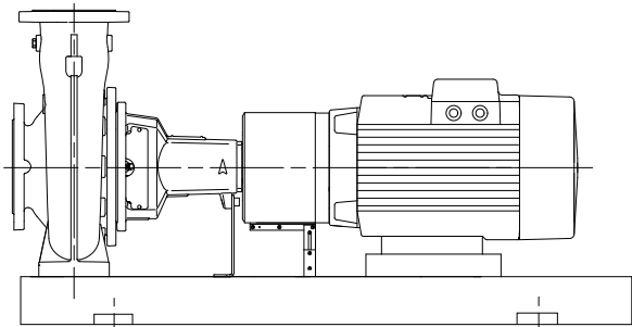
Рис. 64 Насос NKG на плите-основании
