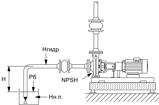
Рис. 40 Высота всасывания воды при положительном значении "Н"
