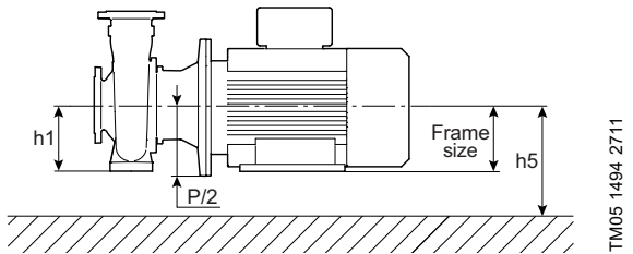
Рис. 71 Обозначение размеров
