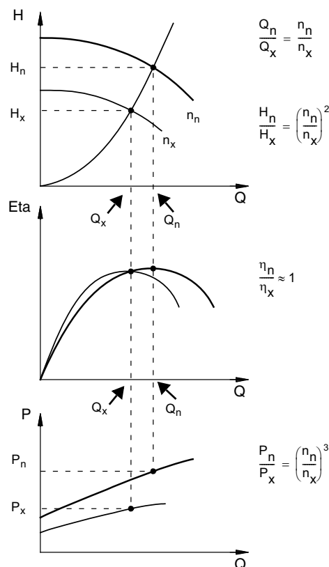
Рис. 57 Уравнения подобия
