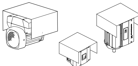
Рис. 51 Вариант дополнительной защиты электродвигателя
