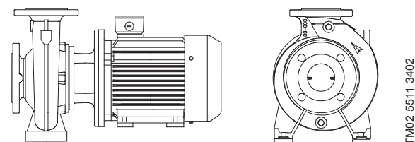
Рис. 12 Исполнение С
