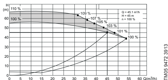
Рис. 48 Расширенный диапазон производительности Е-насосов
