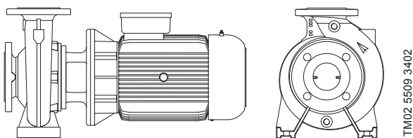
Рис. 10 Исполнение А
