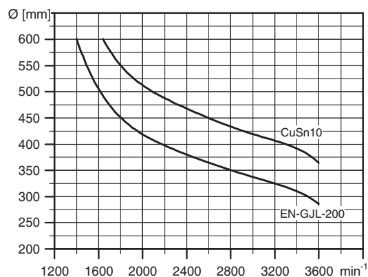
Рис. 49 Максимально допустимая скорость вращения рабочего колеса насоса
