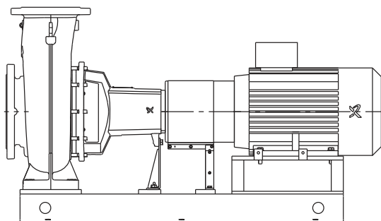
Рис. 58 Насос НК с С-образной плитой-основанием
