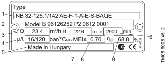
Рис. 5 Пример фирменной таблички
