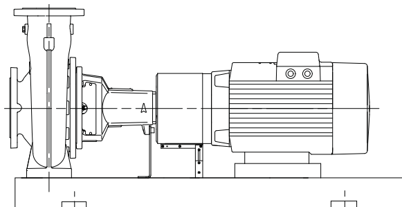
Рис. 57 Насос НК на плите-основании
