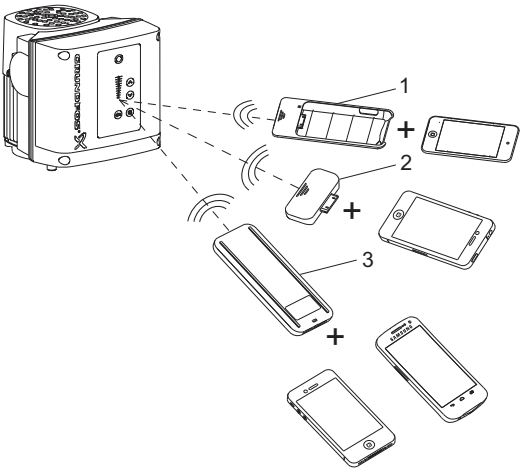
Рис. 54 Связь между GO Remote и насосом посредством радио- или инфракрасного сигнала
