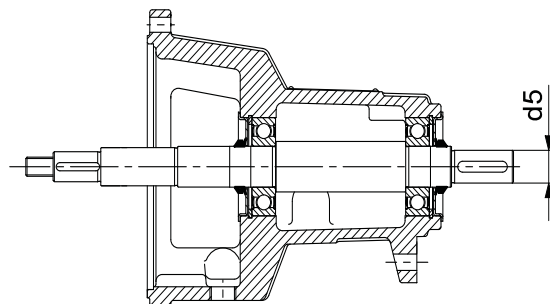
Рис. 15 Кронштейн подшипника и вал
