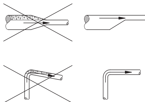
Рис. 42 Трубопроводы
