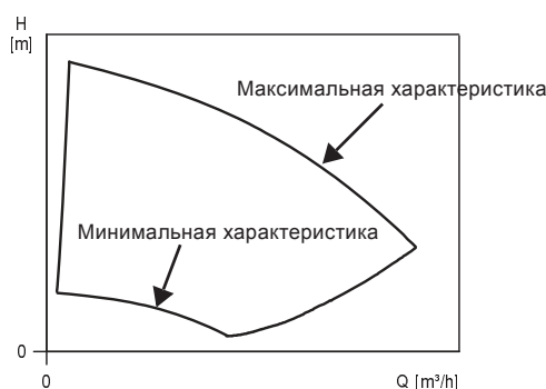
Рис. 50 Мин. и макс. характеристические кривые рабочих точек
