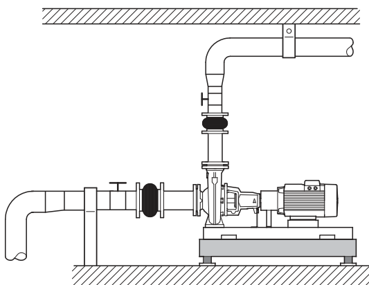
Рис. 43 Монтаж трубопровода
