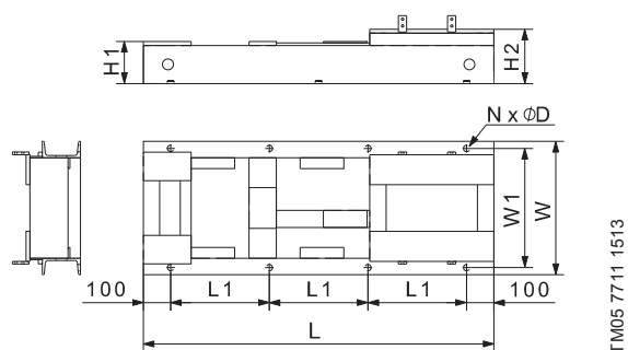
Рис. 61 С-образная плита-основание с 8 установочными отверстиями
