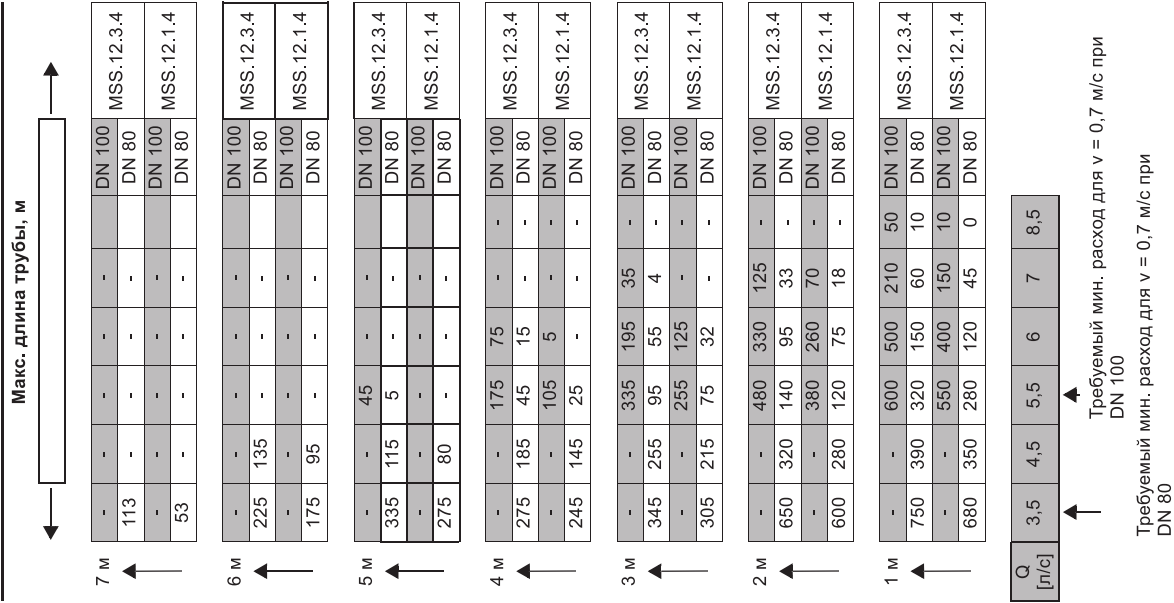
Рис. 86 Максимальная длина вертикальных или горизонтальных напорных трубопроводов
