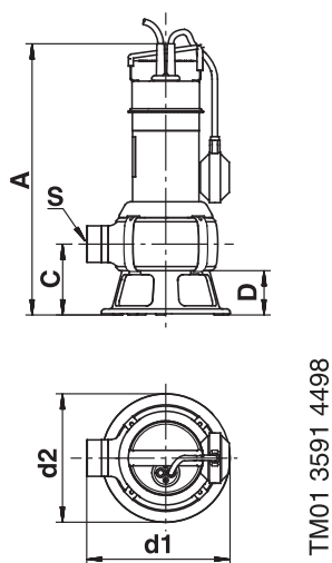
Рис. 31 Габаритные размеры
