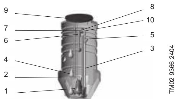
Рис. 138 Пример исполнения колодца.
