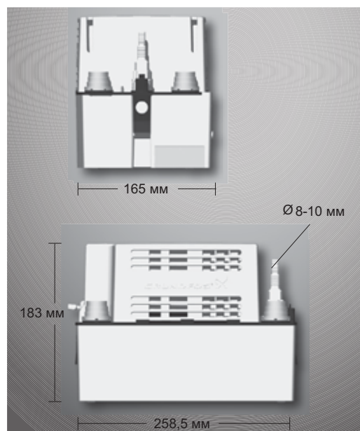
Рис. 72 Габаритные размеры
