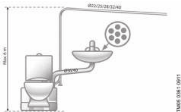
Рис. 38 Для напольного унитаза (Sololift2 WC-1)
