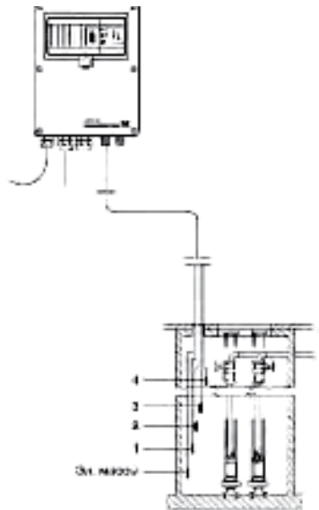
4-х уровневая система для параллельной работы (5 электродов)
