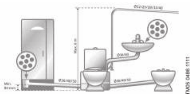
Рис. 39 Для напольного унитаза, раковины, душевой кабины и биде (Sololift2 WC-3)
