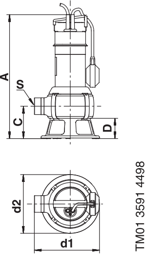
Рис. 29 Габаритные размеры
