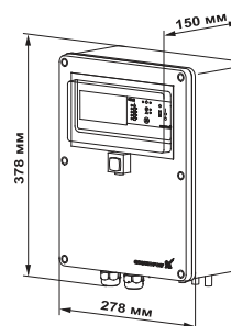
Рис. 122 Габаритные размеры
