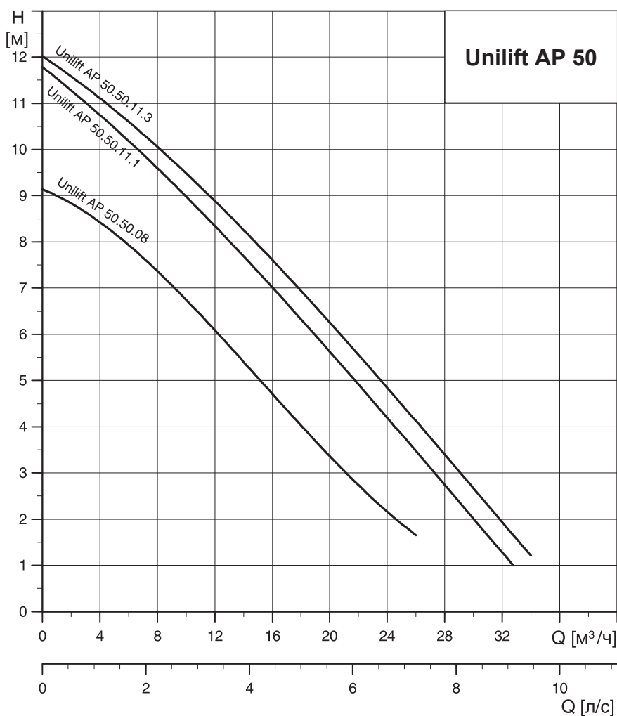
Рис. 23 Кривые характеристик
