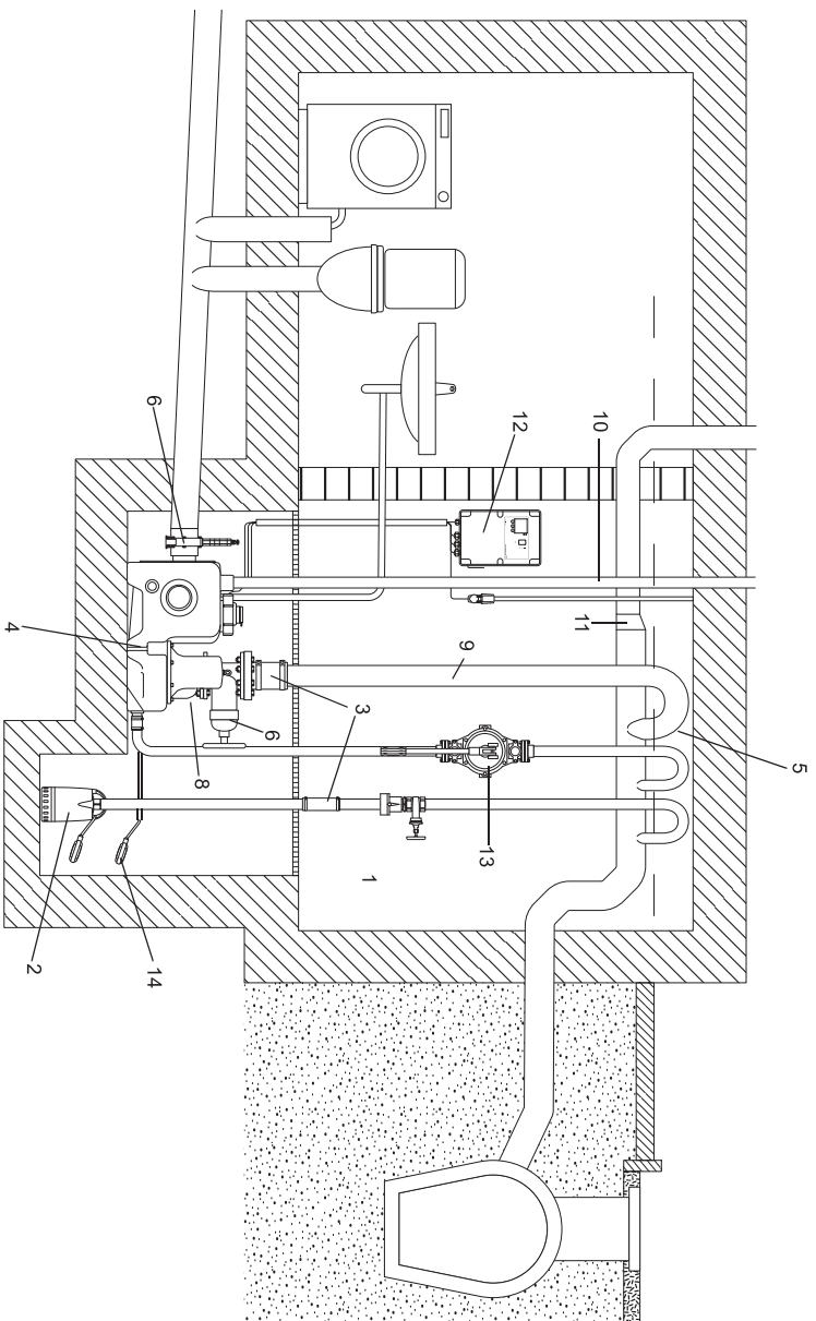
Рис. 82 Пример монтажа насосной установки Multilift
