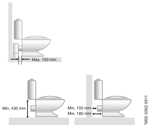
Рис. 36 Обязательные параметры
