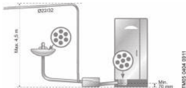
Рис. 41 Для раковины и душевой кабины (Sololift2 D-2)
