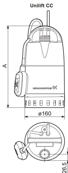
Рис. 3 Габаритные размеры
