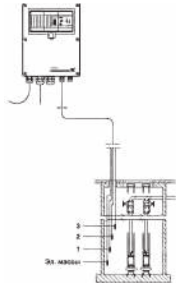
3-х уровневая система для параллельной работы (4 электрода)
