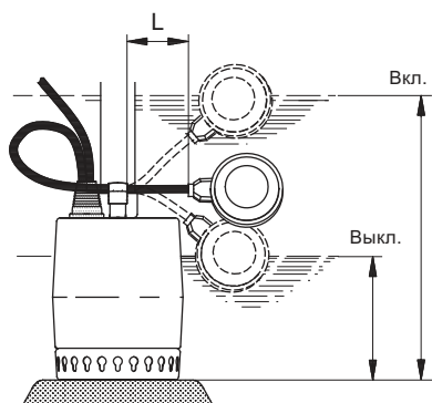
Максимальный и минимальный уровень включения/выключения насоса Unilift KP-A
