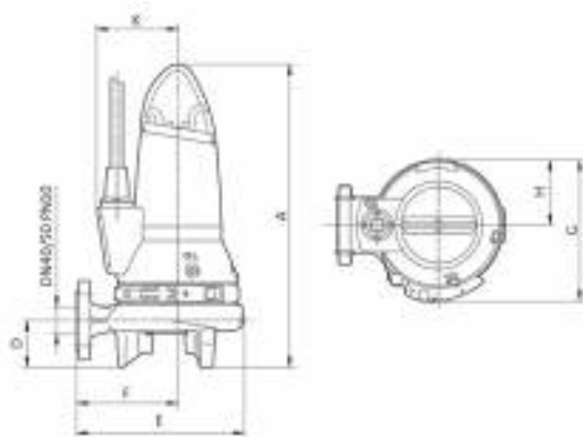
Насос на стандартных опорах
