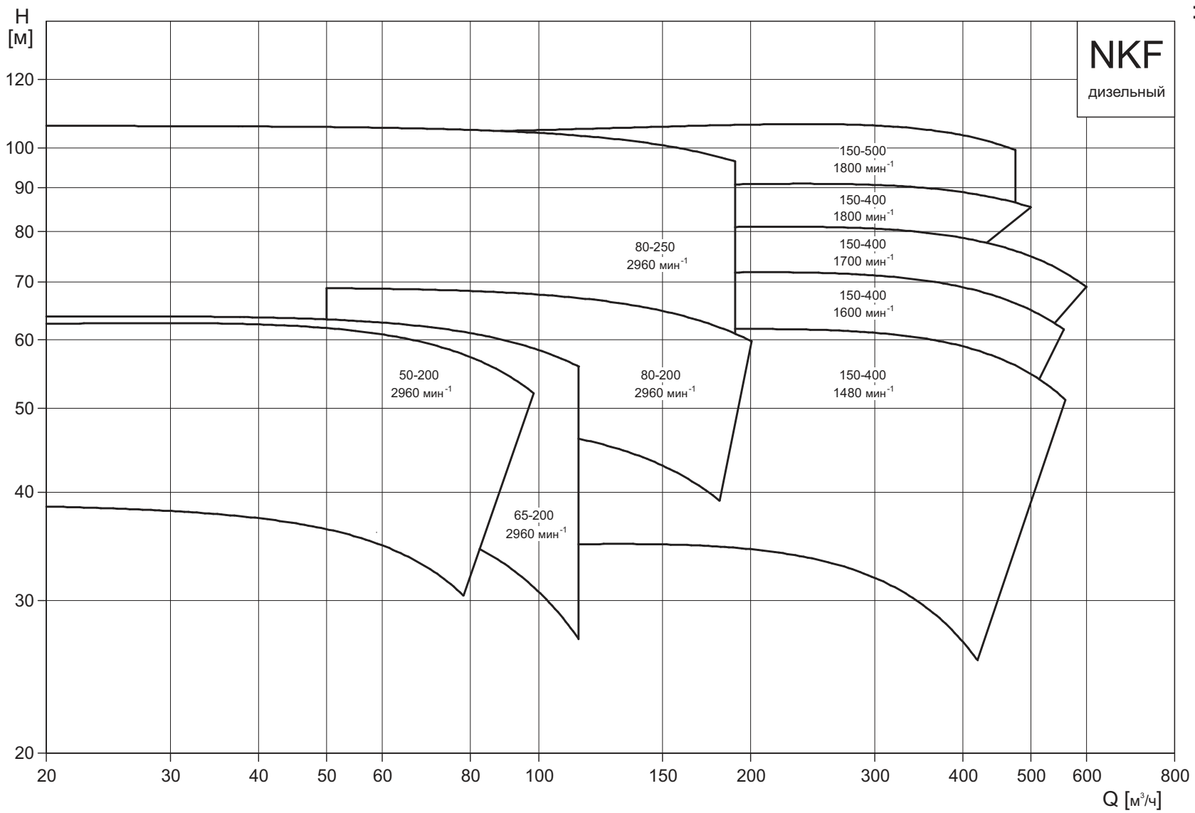
Рис. 15 Графики рабочих характеристик
