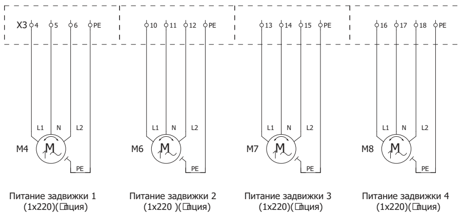
Подключение двигателей 1-фазных задвижек
