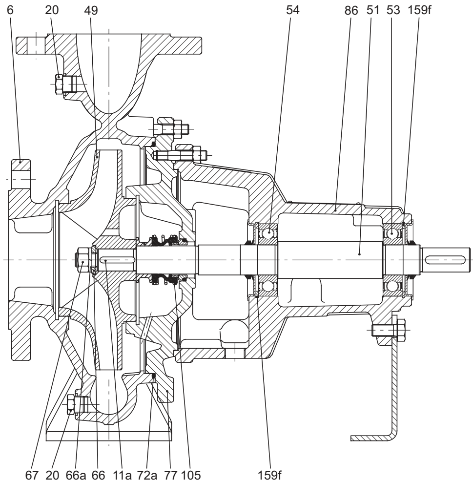
Рис. 17 Чертеж в разрезе NKF 50-200, 65-200, 80-200, 80-250, 150-400, 150-500
