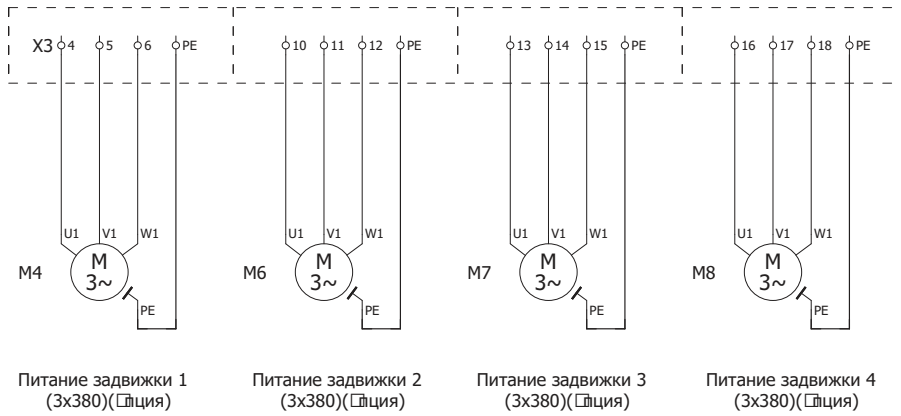
Подключение двигателей 3-х фазных задвижек
