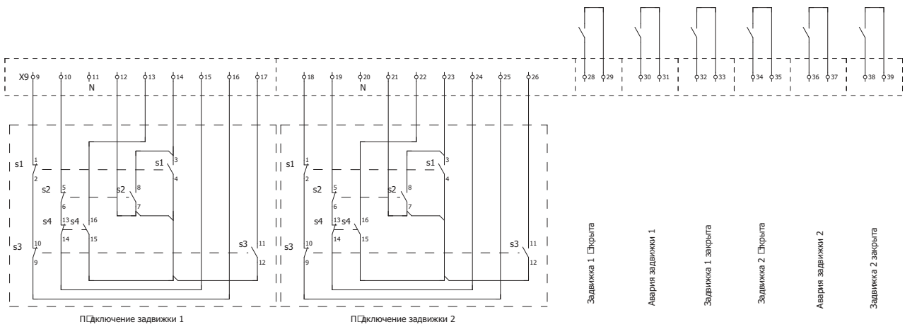
Подключение цепей управления задвижками
