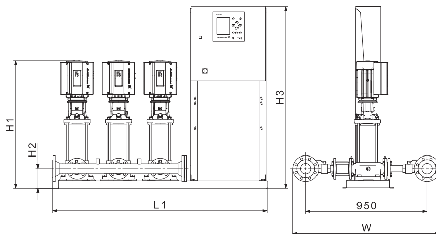
Рис. 39 Размерная схема установки повышения давления Hydro MPC со шкафом управления, который смонтирован на одной раме-основании с насосами (исполнение A). Установка повышения давления приведена в качестве примера. Входящие в поставку насосы могут отличаться от показанных на схеме.
