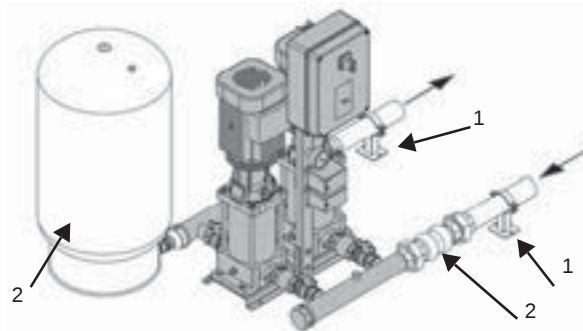
Рис. 3 Пример установки с резиновыми вибровставками и опорами для труб (стандартный объем поставки Grundfos обозначен серым цветом)
