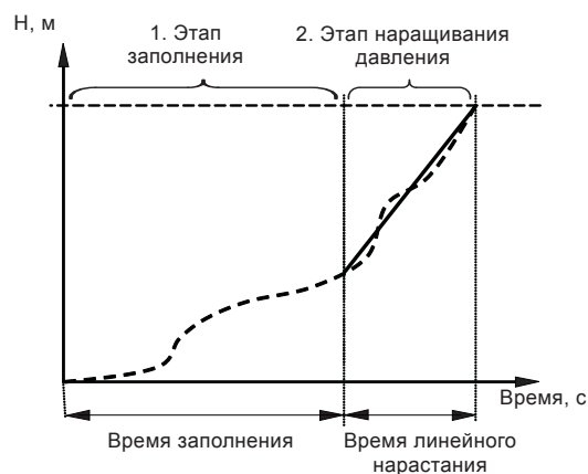
Рис. 31 Этапы заполнения и нарастания давления
