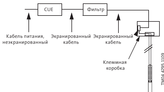
Рис. 3. Пример установки в зонах, чувствительных к радиопомехам
