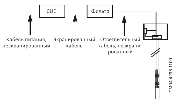
Рис. 2. Пример установки в зонах, не чувствительных к радиопомехам
